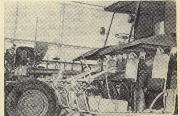
В крупнейшем павильоне ВДНХ СССР будет показан целый арсенал современных машин и механизмов. На снимке: пропалочная машина «ПАУ-4» на базе самоходного шасси «Т-16». Агрегат позволяет повысить производительность труда на самой трудоемкой работе — прополке.
